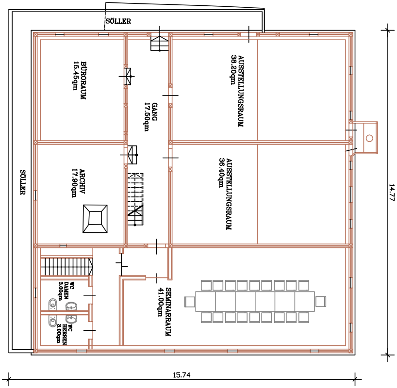
OBERGESCHOSS 1:100
