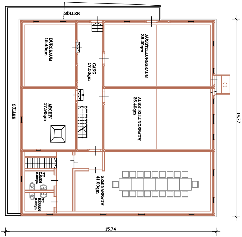
OBERGESCHOSS 1:100
